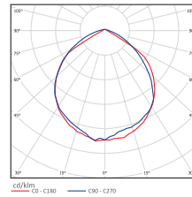
Угол излучения 120°
