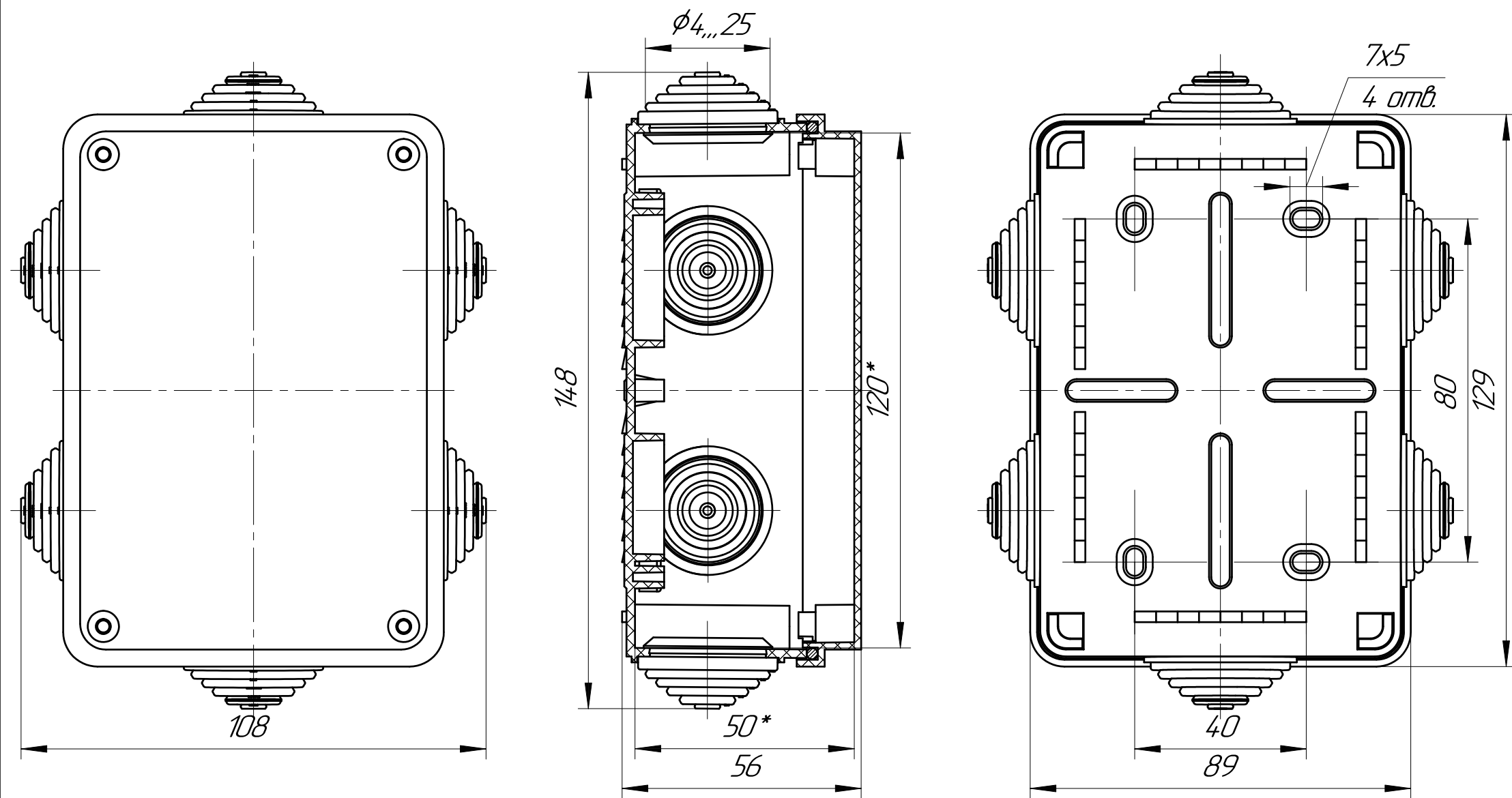
Чертеж 12: Коробка распределительная 40-0340 для о/п безгалогенная (HF) 120x80x50* Промрукав
