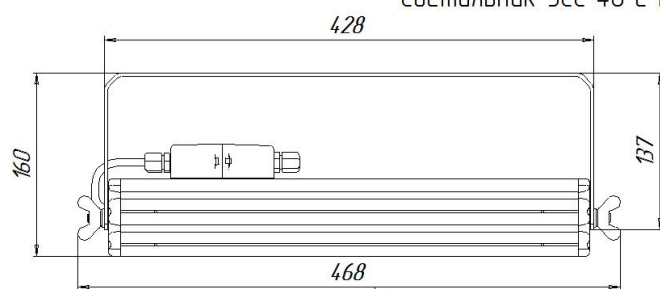
Светильник УСС 48 с креплением скоба
