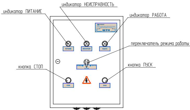
Рисунок 3 - Внешний вид ШУН
