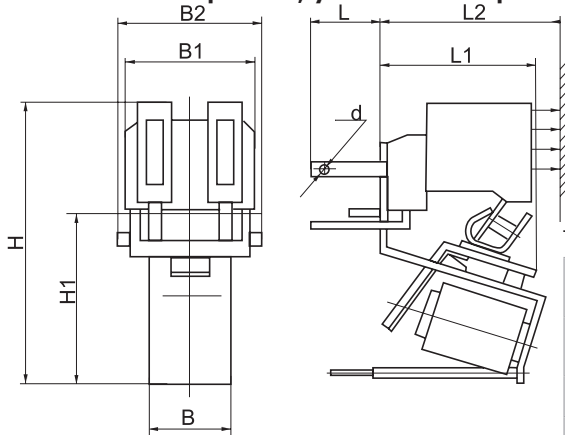
Рисунок В.1. Габаритные и установочные размеры контакторов типа КТПВ-623, КТПВ-624
