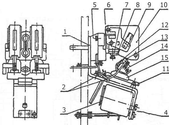
Рисунок 1. Контактор серии КТПВ-620 с двумя замыкающими главными контактами
