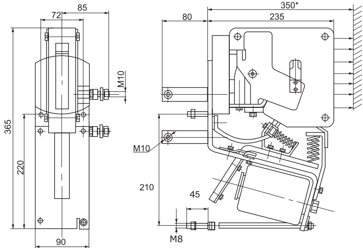
Рисунок В.2. Габаритные и установочные размеры контакторов типа КПВ-604 Масса контакторов КПВ-604 - не более 14,0 кг.
