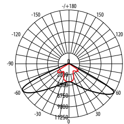
PSL-C-03-150W 5000K 15000Лм
