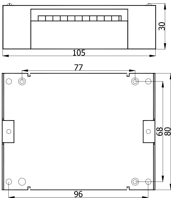
Рисунок 1 Общий вид корпуса.
