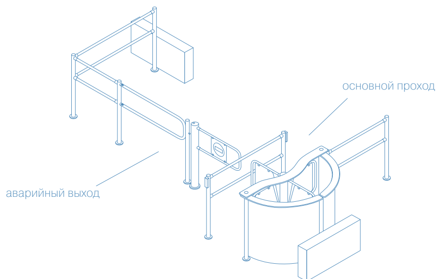
Роторный турникет со стандартными и поворотной секциями ограждений, калитка
