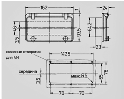
Чертеж 6 MB 12 Размеры, мм.
