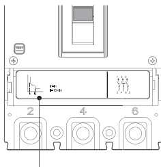
Кривая защиты
