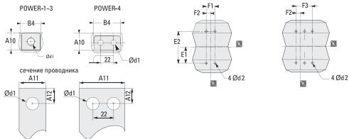
Рис.2 Присоединительные размеры
