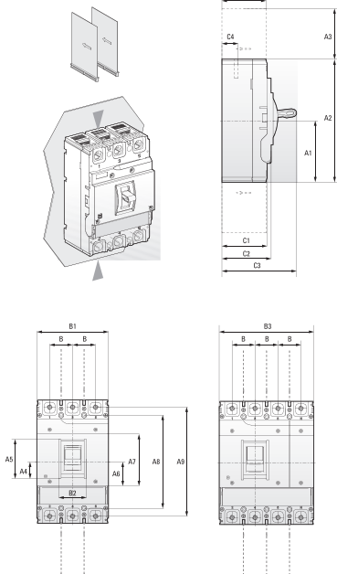
Рис.1 Габаритные размеры выключателя
