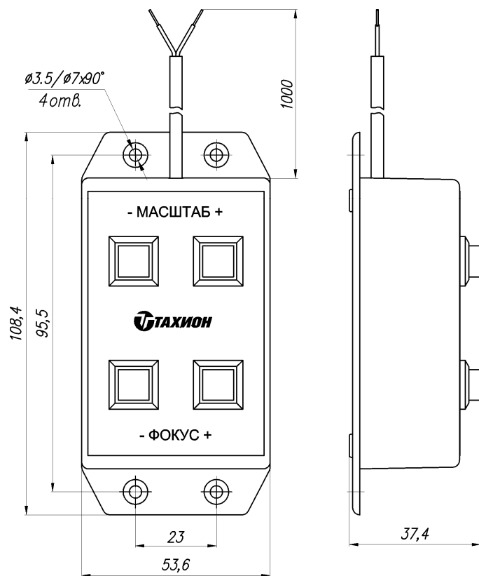
Рис.1 Габаритные размеры
