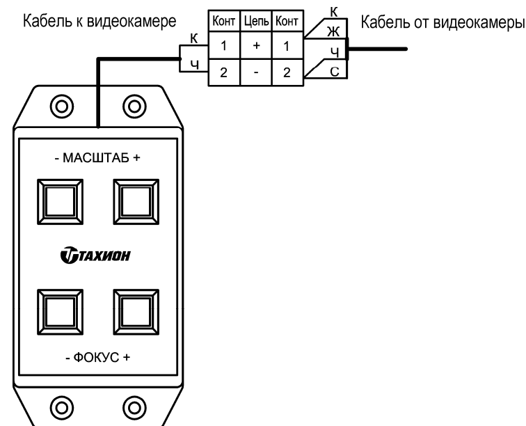
Рис.2 Схема подключения
