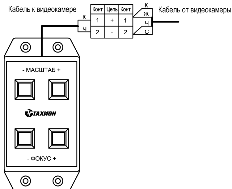
Рис.2 Схема подключения
