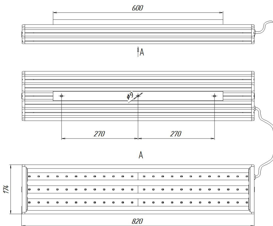
Светильник УСС 130 с 2Ех маркировкой потолочное крепление
