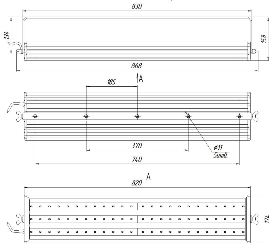
Светильник УСС 130 с 2Ех маркировкой крепление скоба
