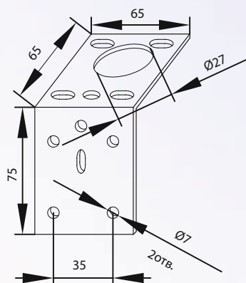
Размеры универсальной скобы подвеса
