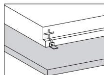
Установка светильников в подшивной потолок на скобы
