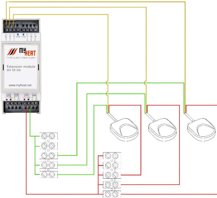
Рис.4. Схема подключения датчика протечки воды к дискретному входу
