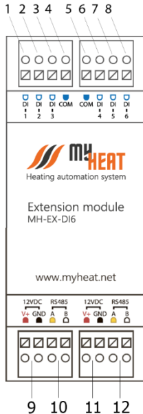
Рис.1. Внешний вид модуля MH-EX-DI6
