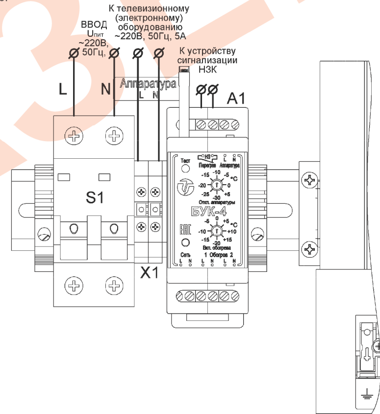
Рис.2. Подключение термощафа
