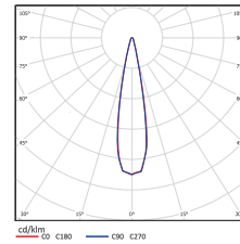
Угол излучения 10°
