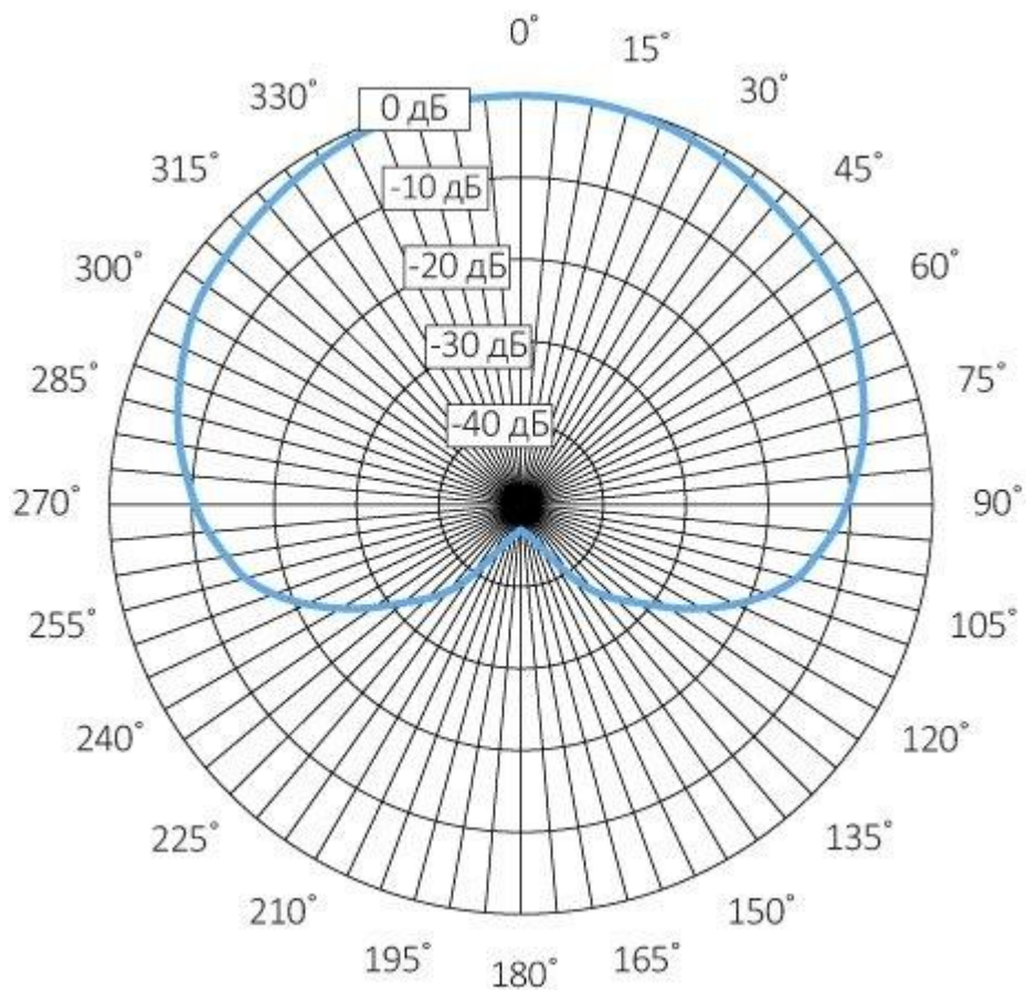
Диаграмма направленности микрофона STELBERRY M-1000 при максимальном значении регулировки
