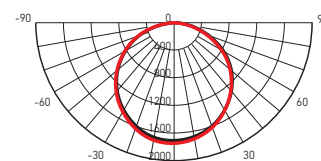
PPL PRO 595/U Prisma 36w
