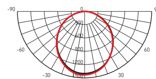
PPL PRO 595/U Opal 36w
