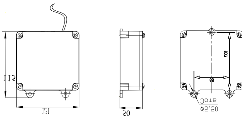
Рис.3 Габаритные и установочные размеры оповещателя ОС-12 «АЯКС» исп.02
