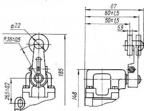
Рис. 4. Выключатели ВП19-21XX31-67X2.XX (остальное см. рис. 2)
