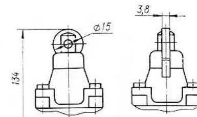
Рис. 6. Выключатели ВП19-21XX22-00X3.XX (остальное см. рис. 5)
