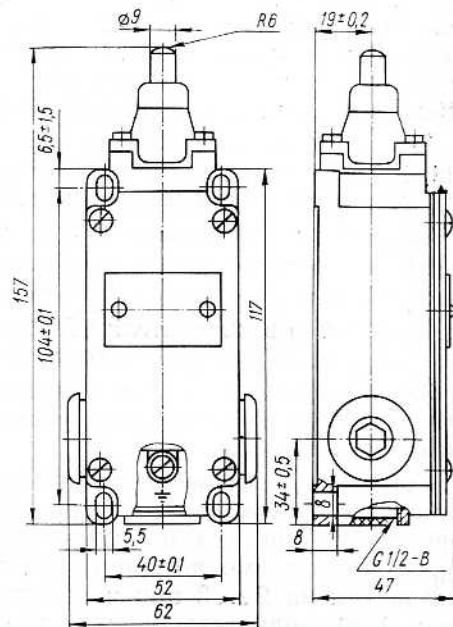
Рис. 2. Выключатель ВП19-21XX11-67X2.XX
