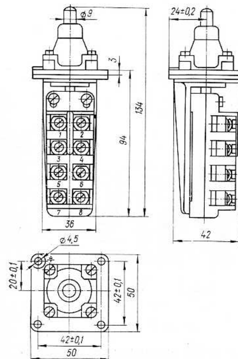
Рис. 5. Выключатели ВП19-21XX12-00X3.XX
