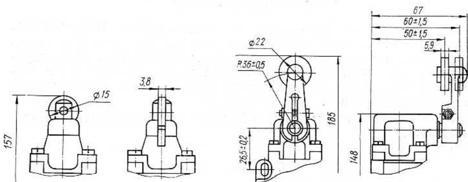
Рис. 3. Выключатель ВП19-21XX21-67X2.XX (остальное см. рис. 2)
