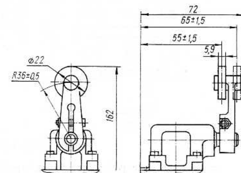
Рис. 7. Выключатели ВП19-21XX32-00X3.XX (остальное см. рис. 5)
