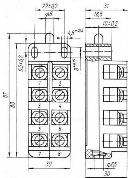
Рис. 1. Выключатель ВП19-21XX11-00X3.XX
