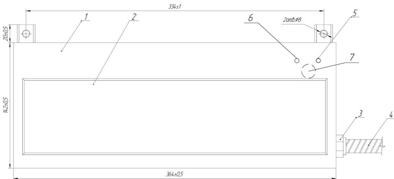
1 корпус; 2 светопропускающее окно; 3 кабельный ввод; 4 кабель питания; 5 индикатор «Сеть»; 6 индикатор режима работы; 7 место расположения магнитного контакта.
