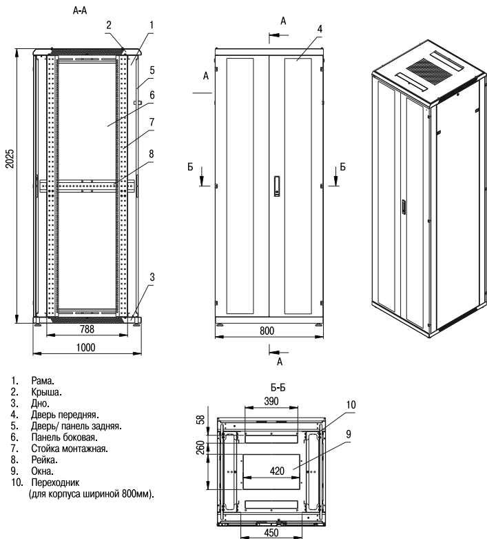
Рисунок 1. Габаритные размеры и внешний вид шкафа
