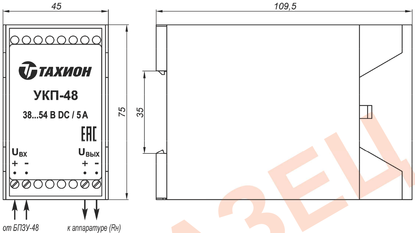
Рис.1 Схема подключения и габаритные размеры УКП-48
