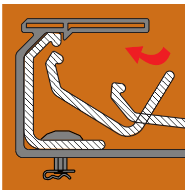
Отрезки соединяются при помощи штифта и без необходимости болтов Поглощает расширения
