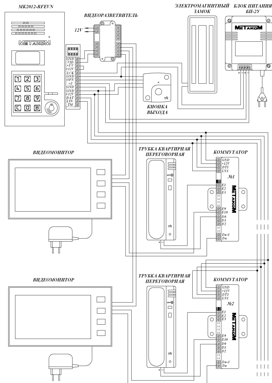
Рис. 2 Пример монтажа блока вызова MK2012-RFEVN
