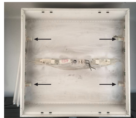
3. Извлекаем старые люминесцентные лампы. Теперь нужно удалить пускатели (стартеры), которые обозначены стрелками.
