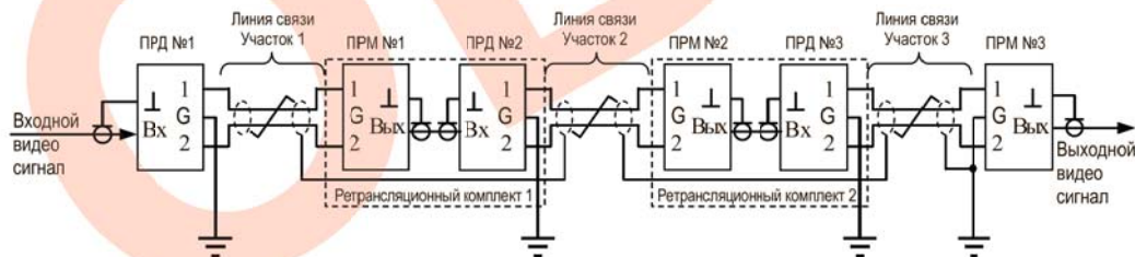
Рис.6 Схема построения линии связи с max длиной 4,8 км, состоящей из трёх участков
