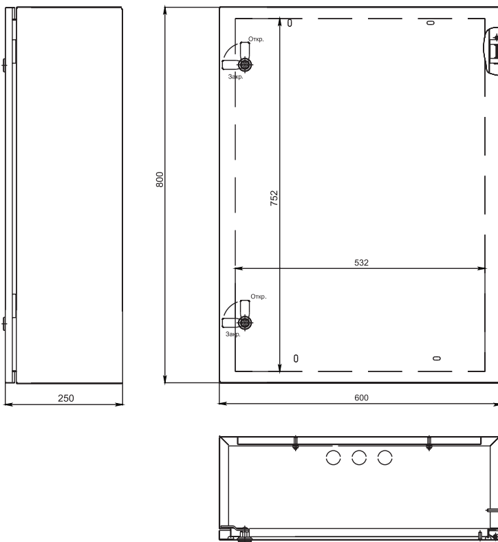
ЩМПГ-80x60x25
