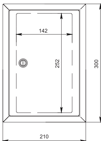
ЩМП-30x21x14
