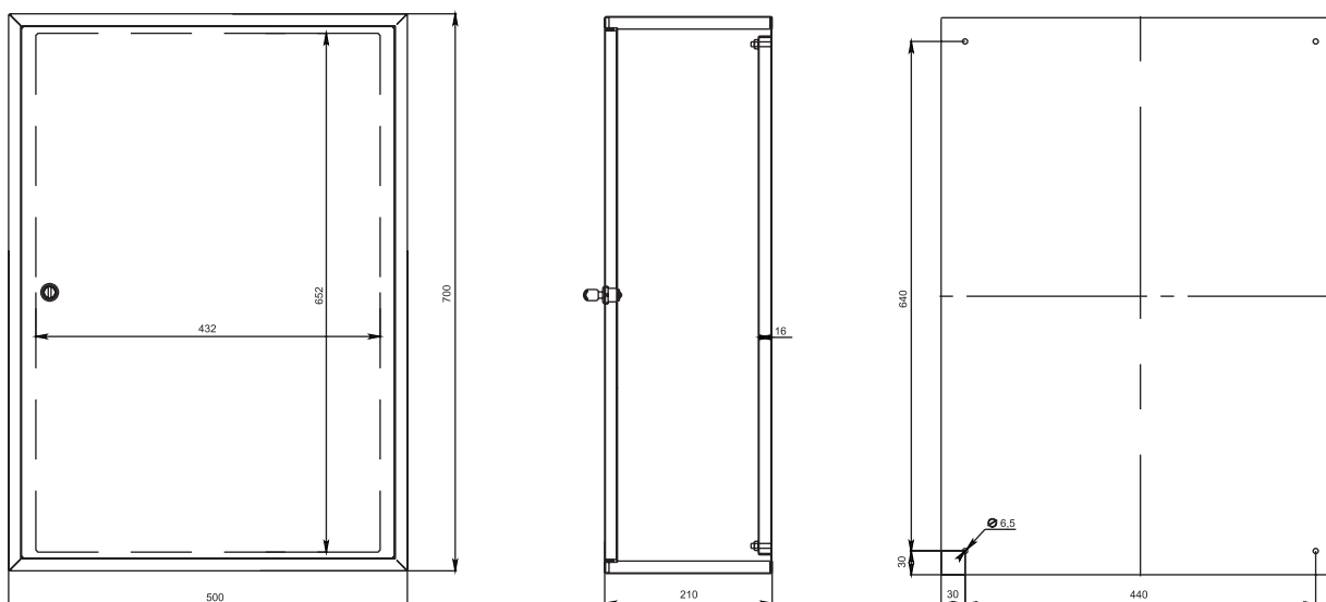
ЩМП-70x50x21
