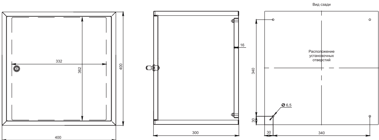
ЩМП-40x40x30
