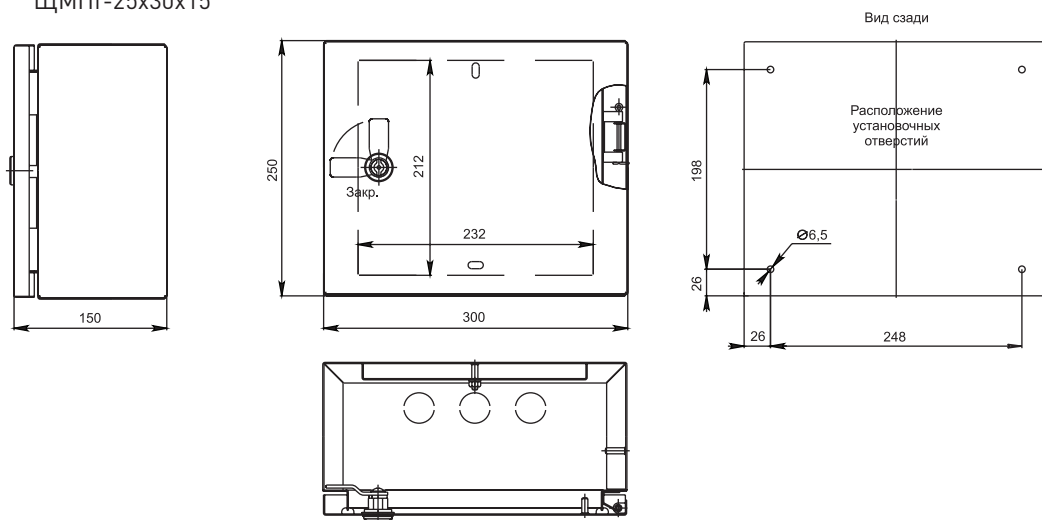
ЩМПГ-25x30x15
