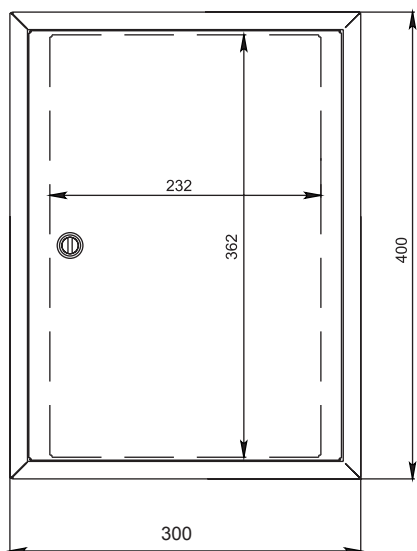
ЩМП-40x30x15
