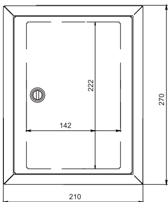
ЩМП-27х21х14
