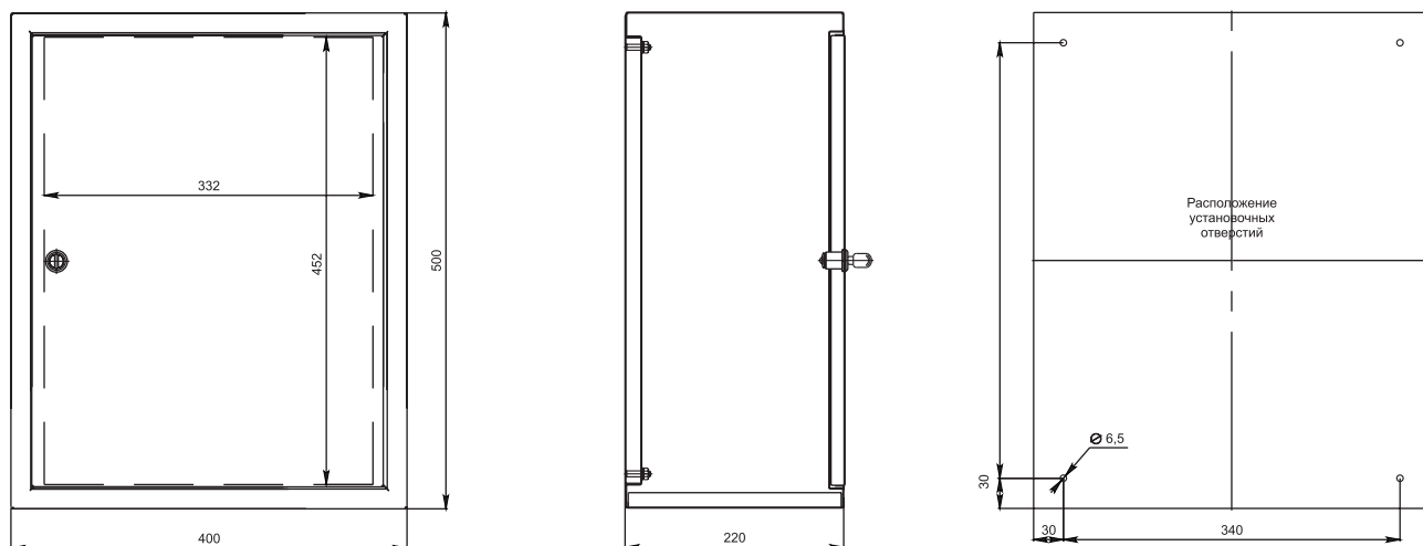
ЩМП-50x40x22
