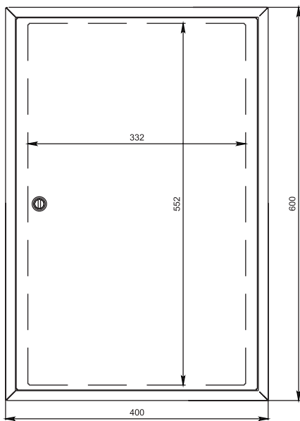
ЩМП-60x40x40 (ЩМП-11)
