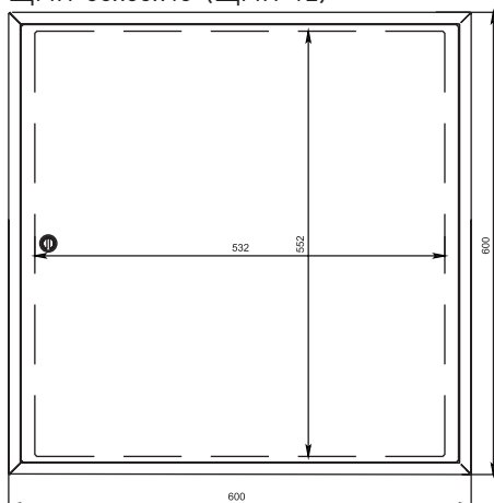
ЩМП-60x60x40 (ЩМП-12)
