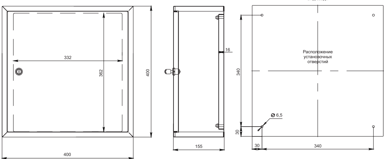
ЩМП-40x40x15
