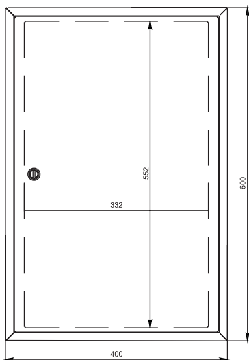
ЩМП-60x40x40 (ЩМП-11)
