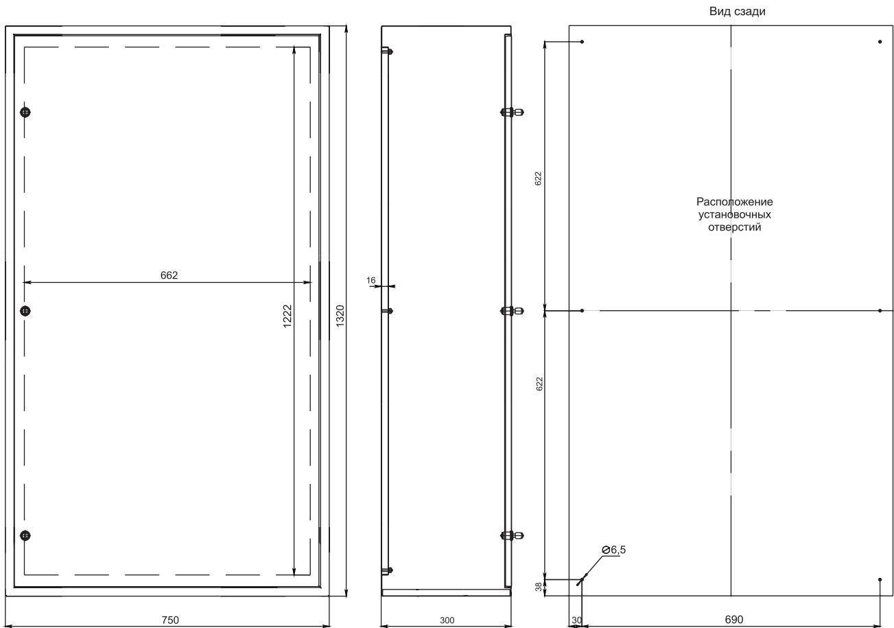
ЩМП-132x75x30
