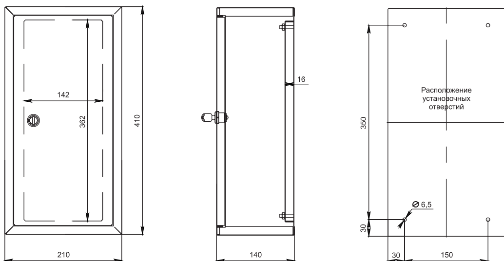
ЩМП-50x40x17
