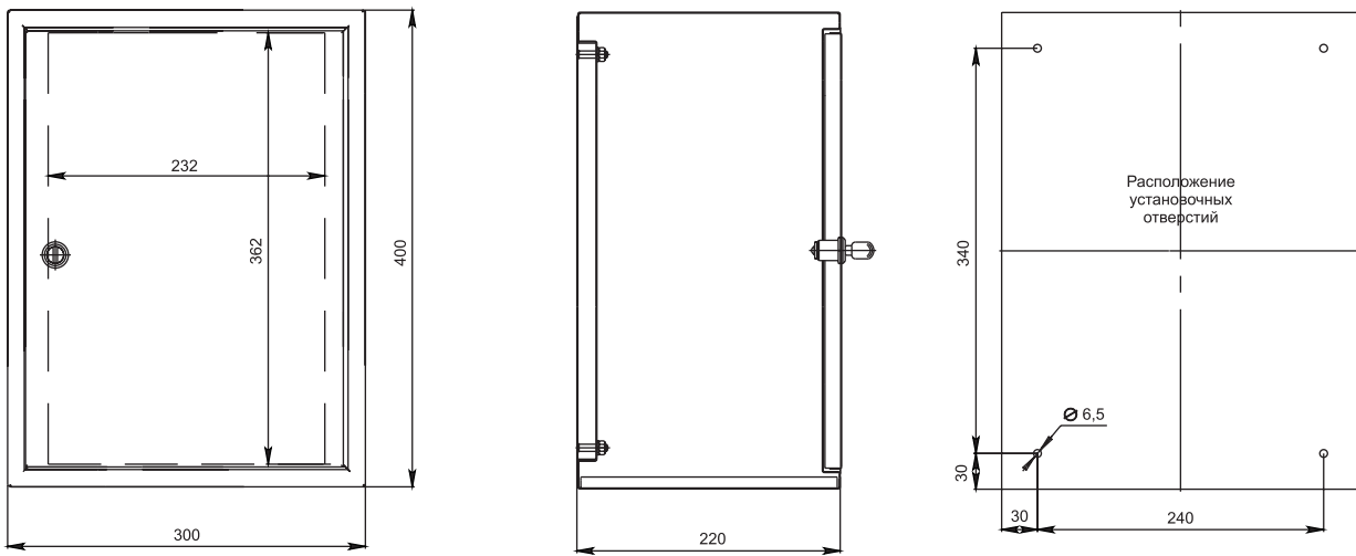
ЩМП-40.30.22
