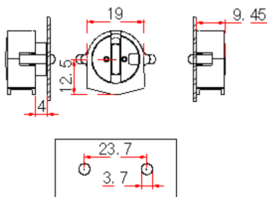
Патрон (ламподержатель)G5 торцевой, встраиваемый в 9,4мм для люминесцентной лампы Т5, без пружины (крепление на цапфы)
