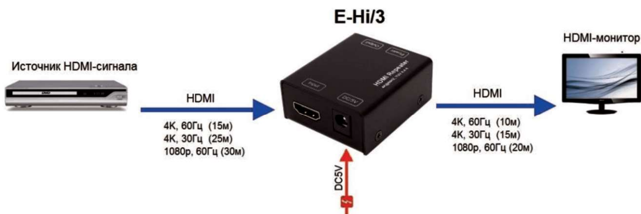
Рис.3 Схема подключения E-Hi/3
