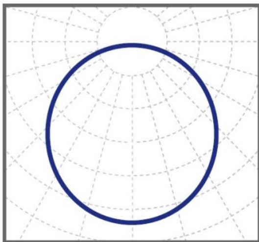
косинусная Д КСС 115°
