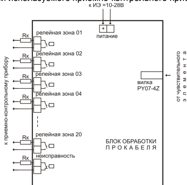
Рис.6. Внешние соединения блока обработки извещателя.
