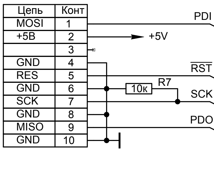
Рис.П.Б.1 – Контакты разъёма «PRG» БО для подключения программатора.
