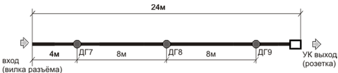
Рис.2. Расположение газовых датчиков (ДГ) в кабельном хвосте ИПГМ.
