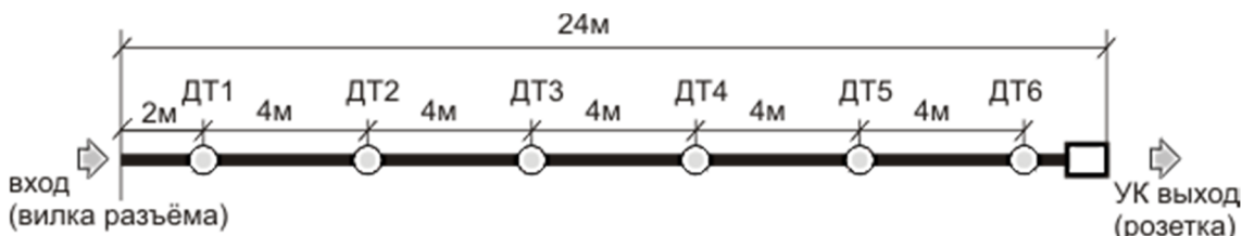
Рис.1. Расположение тепловых датчиков (ДТ) в кабельном хвосте ИПТМ.
