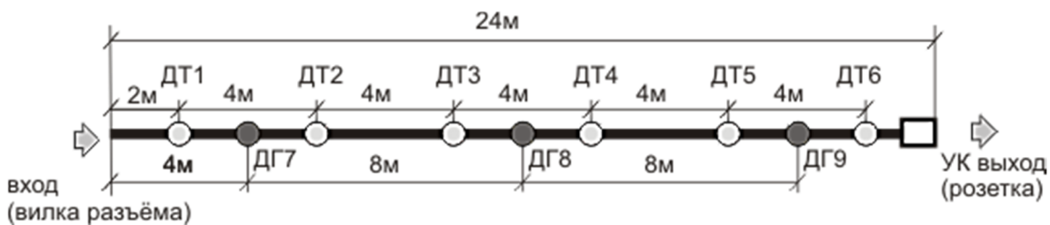
Рис.3. Расположение тепловых датчиков (ДТ) и газовых датчиков (ДГ) в кабельном хвосте ИПКМ (газ, тепло).
