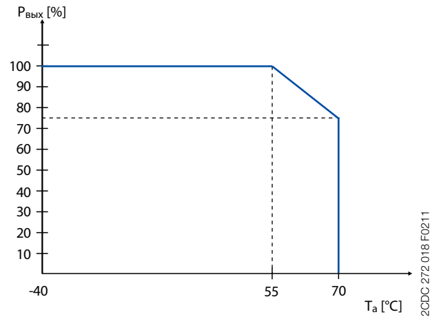
CP-E 24/20.0, CP-E 48/10.0
