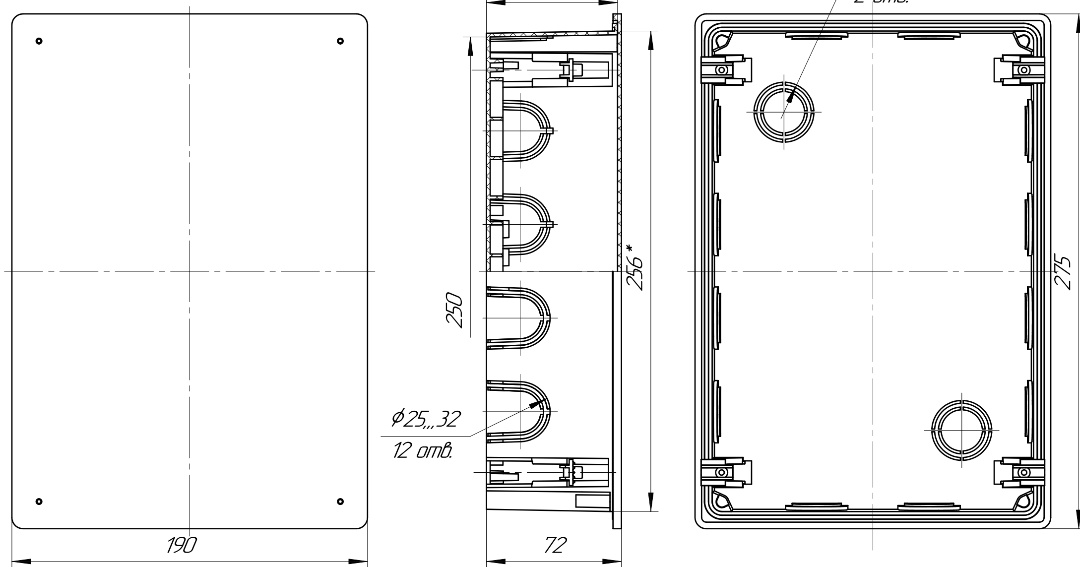
Чертеж 18: Коробка распределительная 80-0980 для о/п безгалогенная (HF) 256x171x70* Промруков
