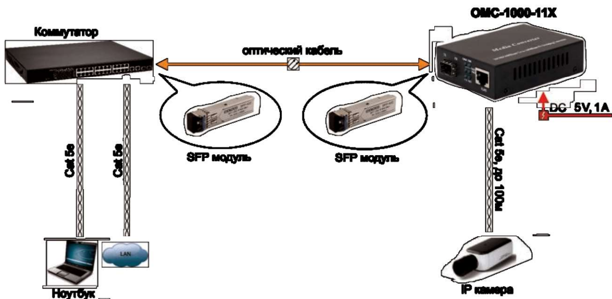
Рис.5 Типовая схема подключения медиаконвертера OMC-1000-11X
