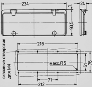
Чертеж 6 МВ 14 Размеры, мм.
