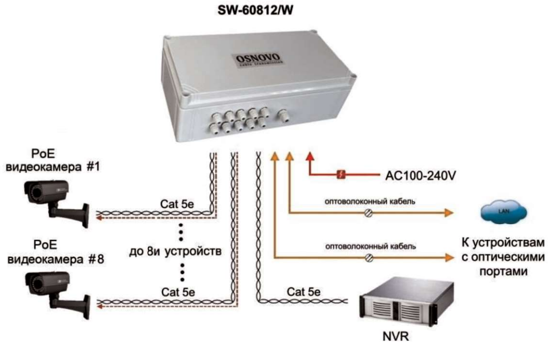
Рис.6 Типовая схема подключения коммутатора SW-60812/W
