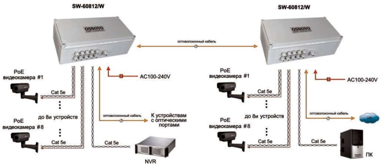
Рис.7 Схема каскадного подключения коммутатора SW-60812/W
