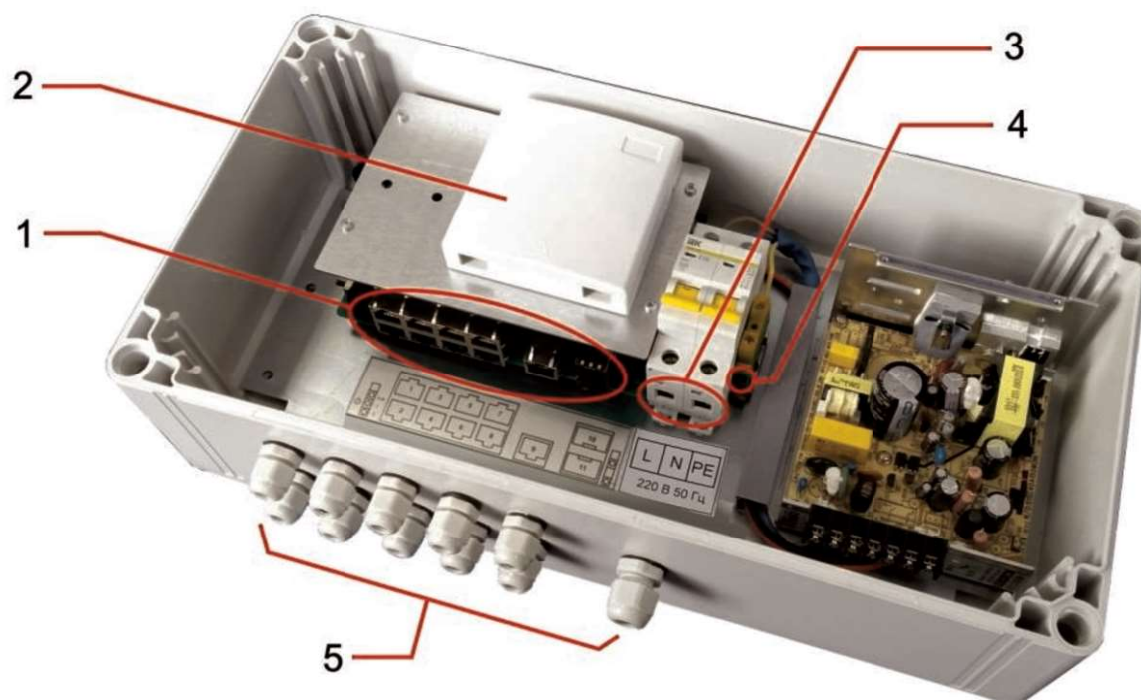
Рис. 2 Коммутатор SW-60812/W, вид внутри
