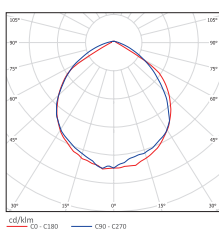
Угол излучения 120°
