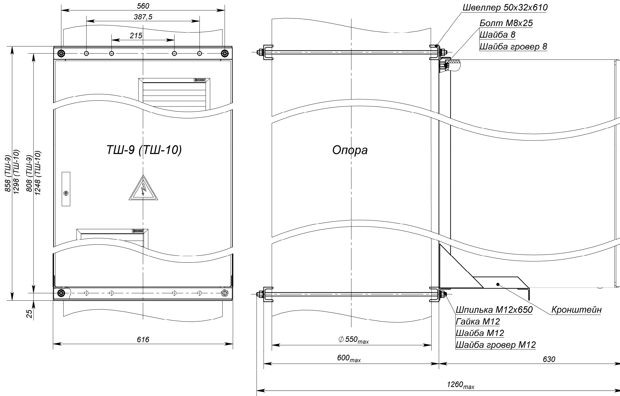
Рис.2 Габаритные и установочные размеры крепления на опору ТШ-9 (ТШ-10)
