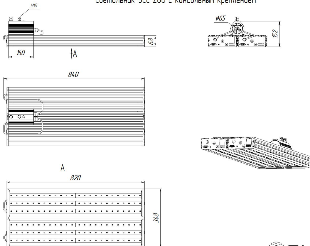
Светильник УСС 260 с консольным креплением
