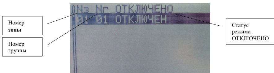
Рис.12 Меню ОТКЛЮЧЕНО, вызывается кнопками «F2»-«8» (расшифровки направлений поступления сигнала ОТКЛЮЧЕНО).
