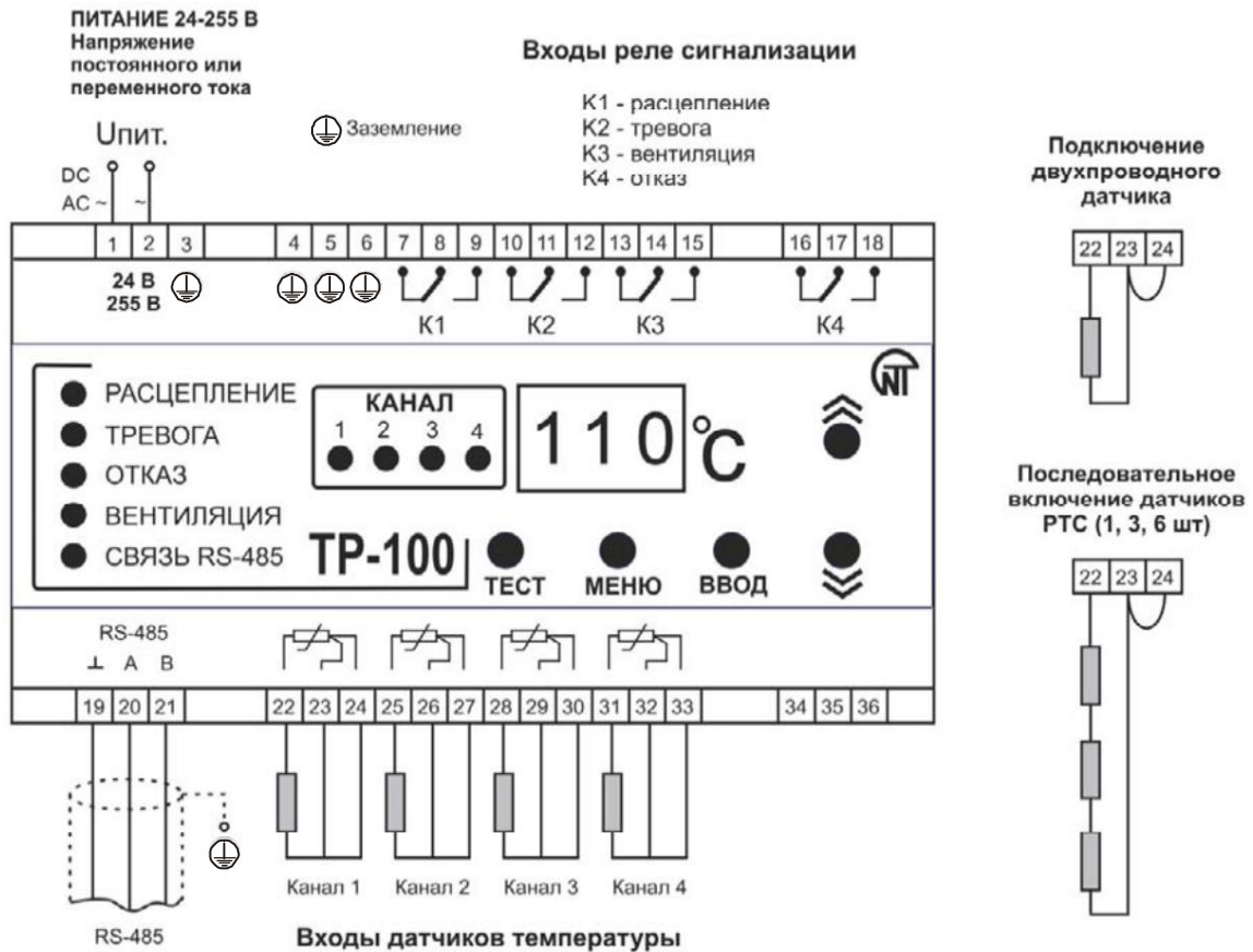
Рисунок 2 – Электрические соединения TP-100
