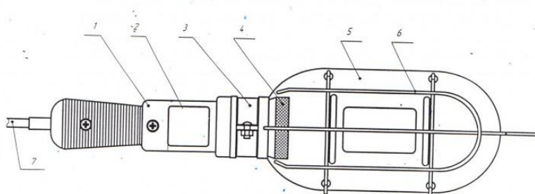
Переносной светильник типа РВО
