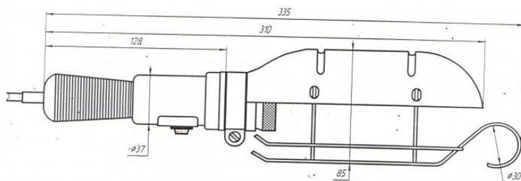
Основные габаритные размеры переноски.
