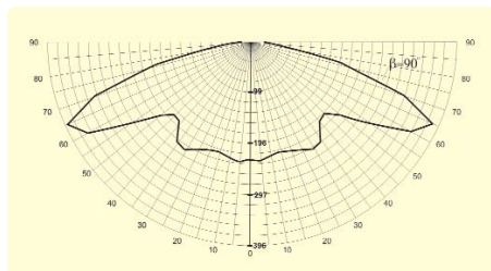
ЖКУ 66-250-002 со стеклом угол 90°
