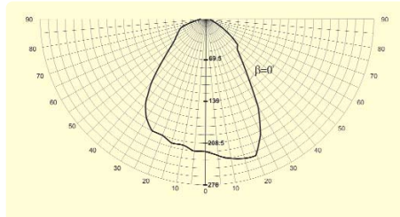
ЖКУ 66-150-003 без стекла угол 0°
