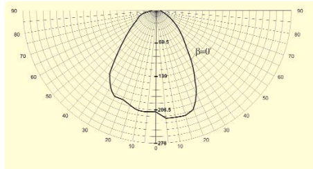
ЖКУ 66-150-002 с плоским стеклом угол 0°
