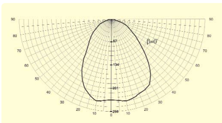
ЖКУ 66-250-002 со стеклом угол 0°
