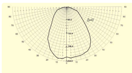
ЖКУ 66-250-003 без стекла угол 0°
