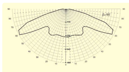
ЖКУ 66-250-003 без стекла угол 90°
