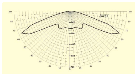
ЖКУ 66-150-003 без стекла угол 90°
