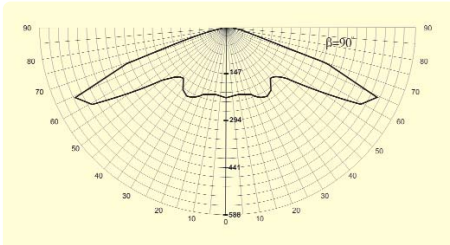
ЖКУ 66-150-002 с плоским стеклом угол 90°
