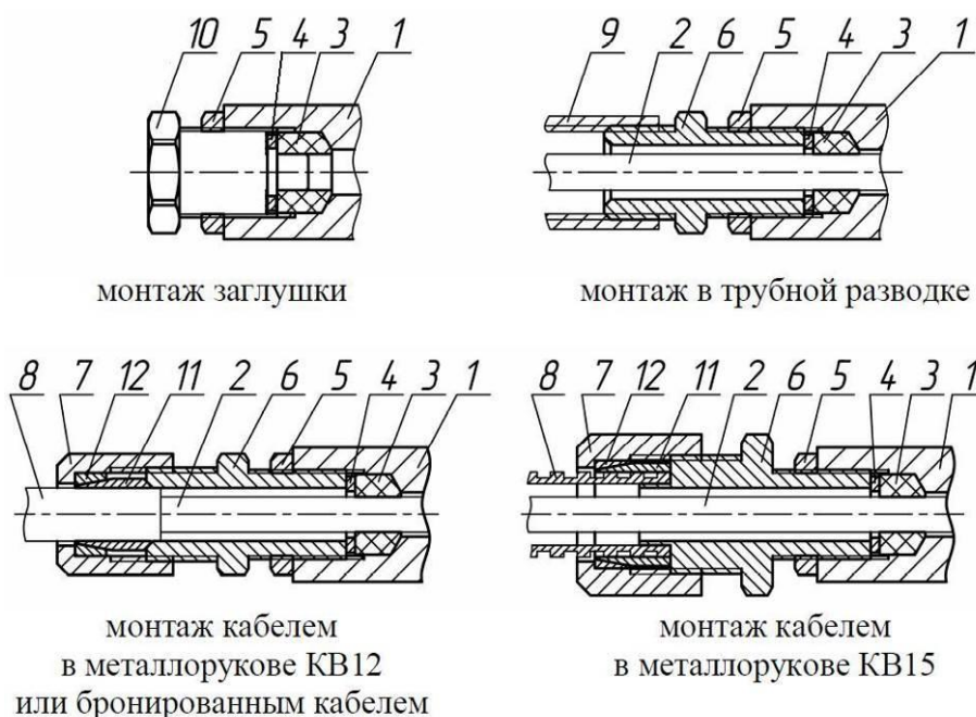
Рисунок 10 – Различные вводные устройства
