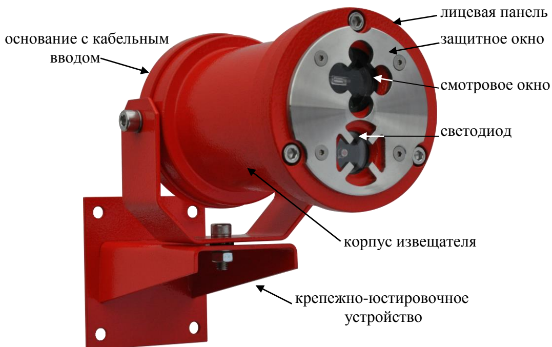
Рисунок 2 – Внешний вид извещателя
