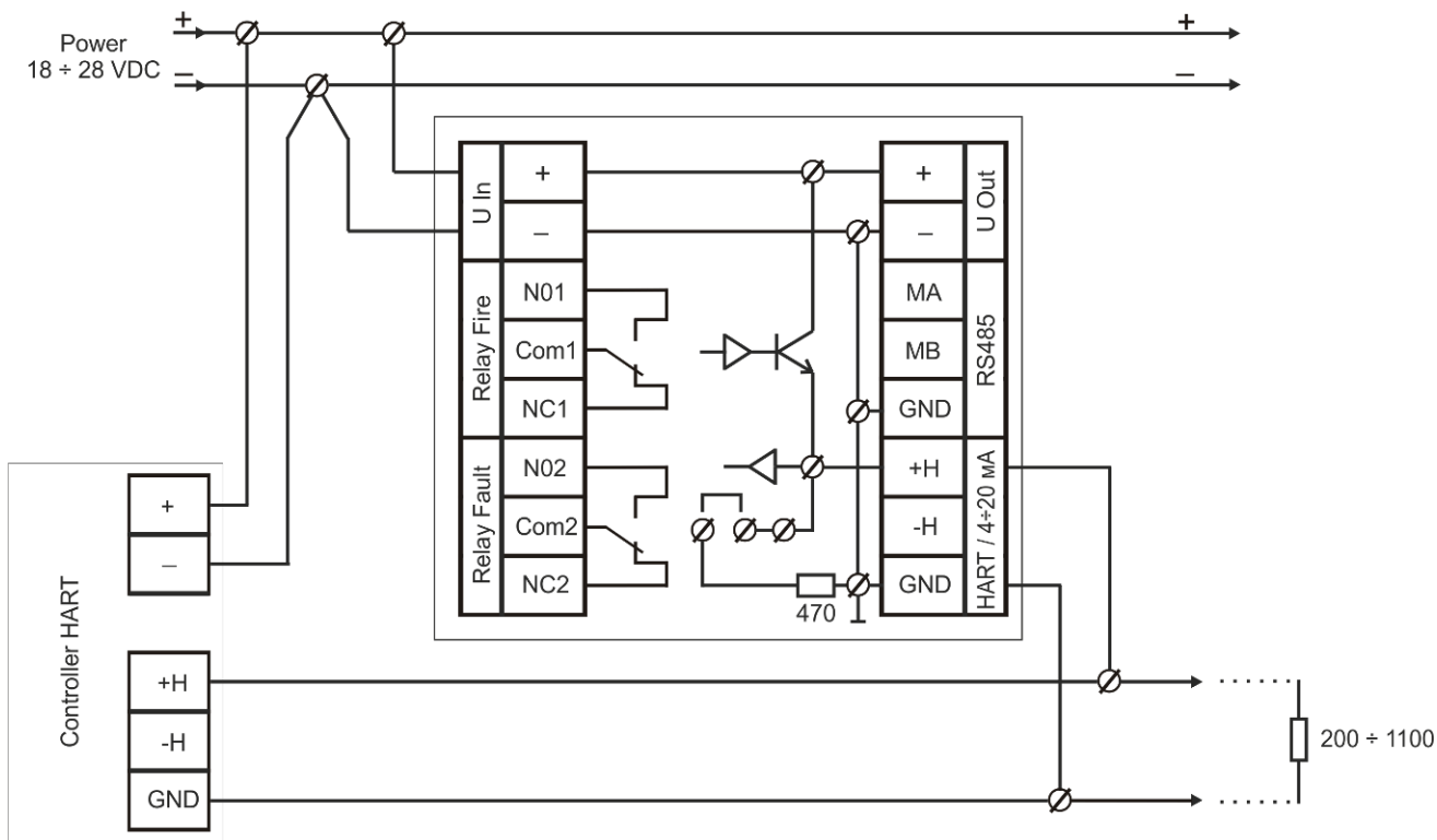
Рисунок 7 – Схема подключения по интерфейсу HART
