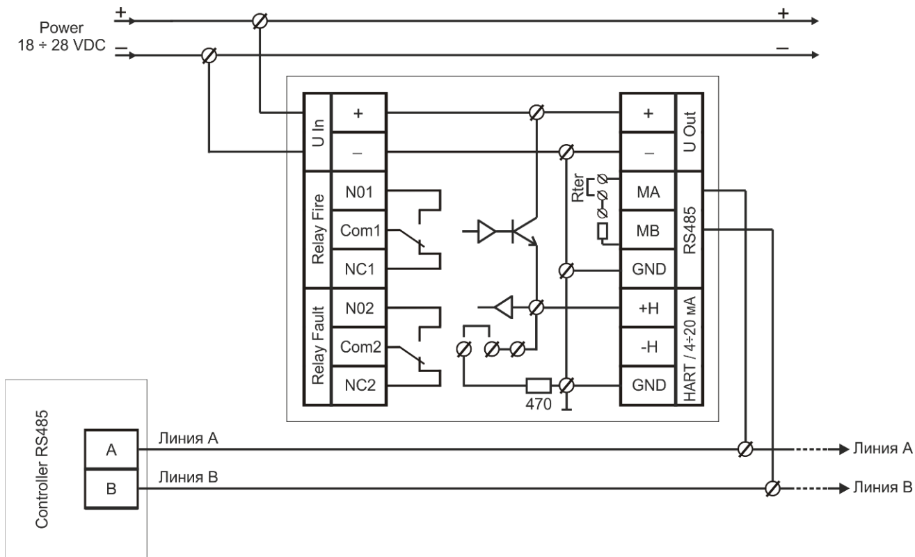
Рисунок 8 – Схема подключения по интерфейсу RS485
