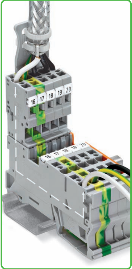
Экранирующая передача (на рисунке показан соединитель X-COM)
