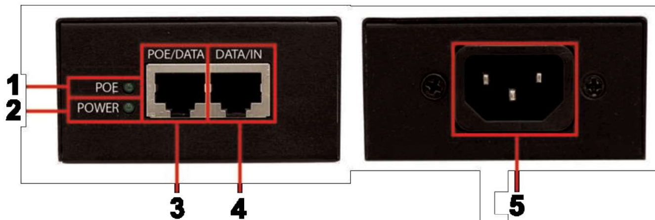
Рис. 2 Midspan-1/652G, разъемы на передней и задней панелях
