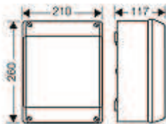
Чертеж с размерами
