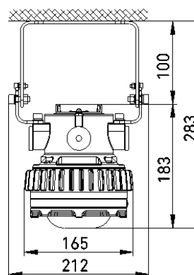
Потолочный
