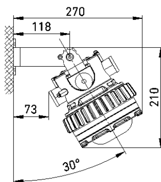
Настенный, 30°
