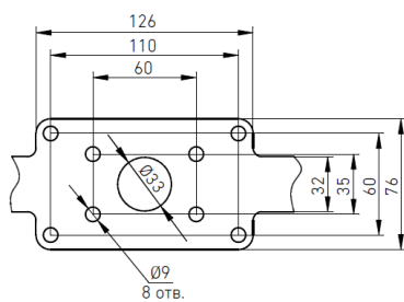
УСТАНОВОЧНЫЕ РАЗМЕРЫ СКОБ
