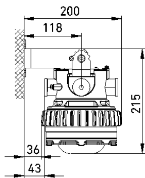
Настенный, 90°
